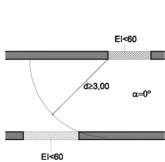
Figura 1.1. Fachadas enfrentadas
