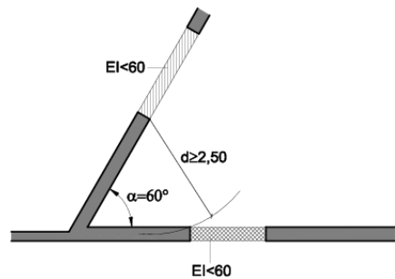
Figura 1.3. Fachadas a 60°
